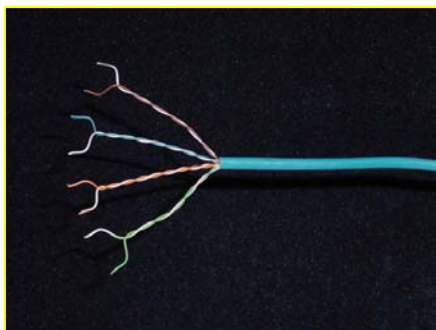
CAT-5
